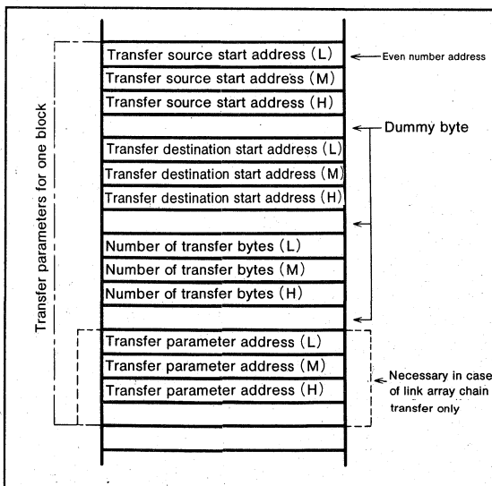
Fig.67 Parameter memory format
